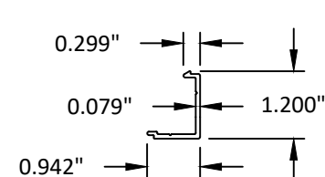
31 1 1/4\" X 1\" CLIP 6063-T5
