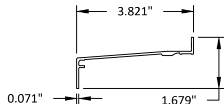
8 3\" SILL TRIM 6063-T5
