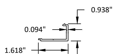
39 MULLION CLIP 6063-T5
